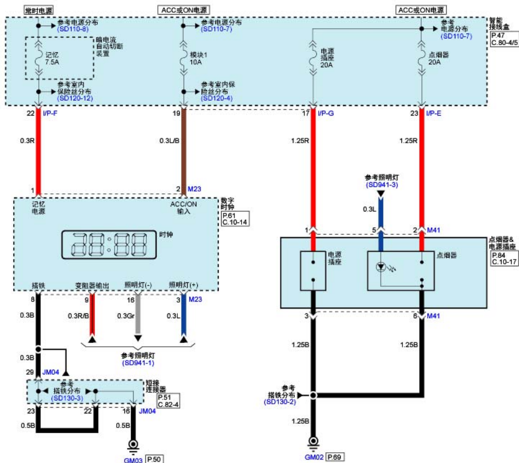
时钟&amp;点烟器(电源插座)系统(2)
